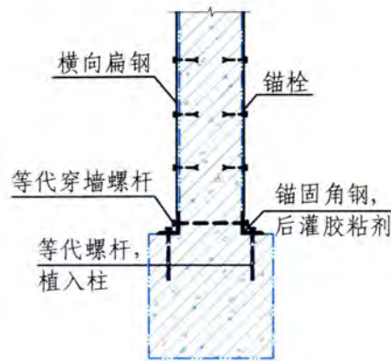
双面加固(一)
