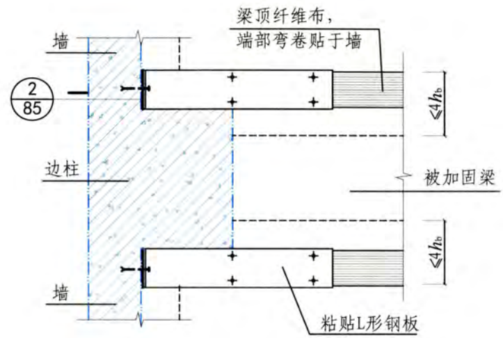
3-3 (梁顶有柱有墙时, L形钢板锚固)
