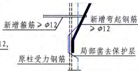
新增弯起钢筋与原柱筋焊接
