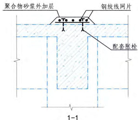
(梁顶无障碍时)
