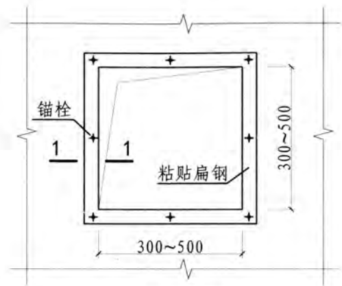
方形洞
