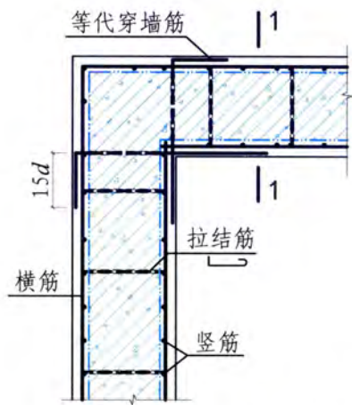
纵横墙双面加固
