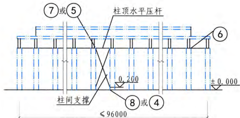
2-2 (非抗震区及6、7度设防区)
