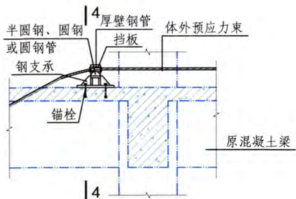
4 转向块4
