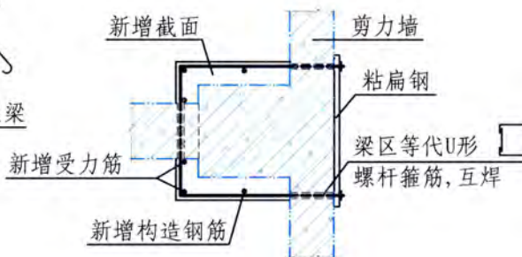
6-6
