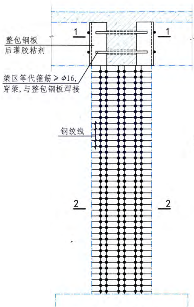
钢绞线横向布置详图
