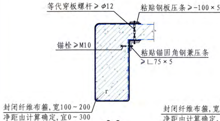
2-2 (加锚封闭箍)
