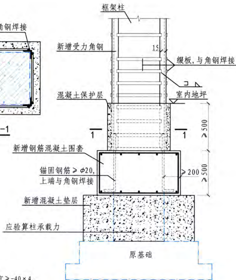
新增钢筋混凝土围套锚固
