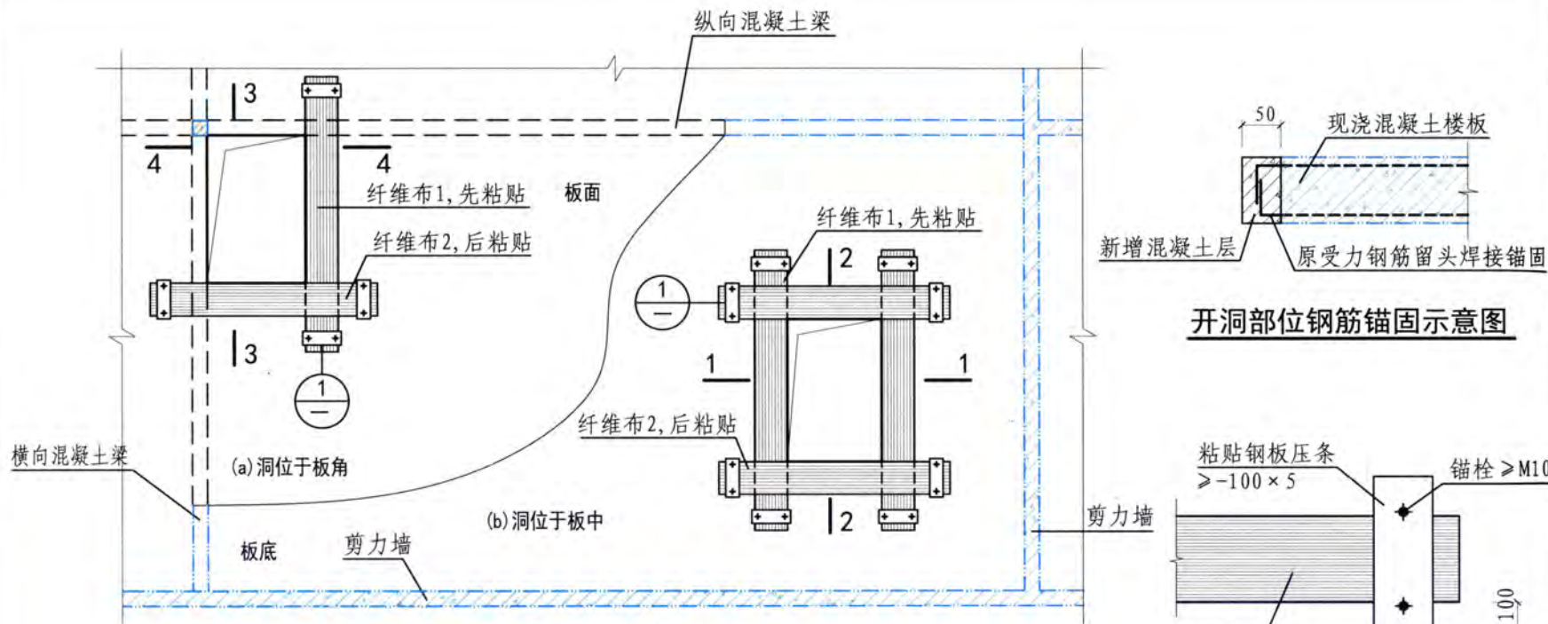
粘贴纤维布补偿加固现浇板开洞 (俯视/仰视)
