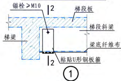
梁式楼梯梯梁加固 (二)
