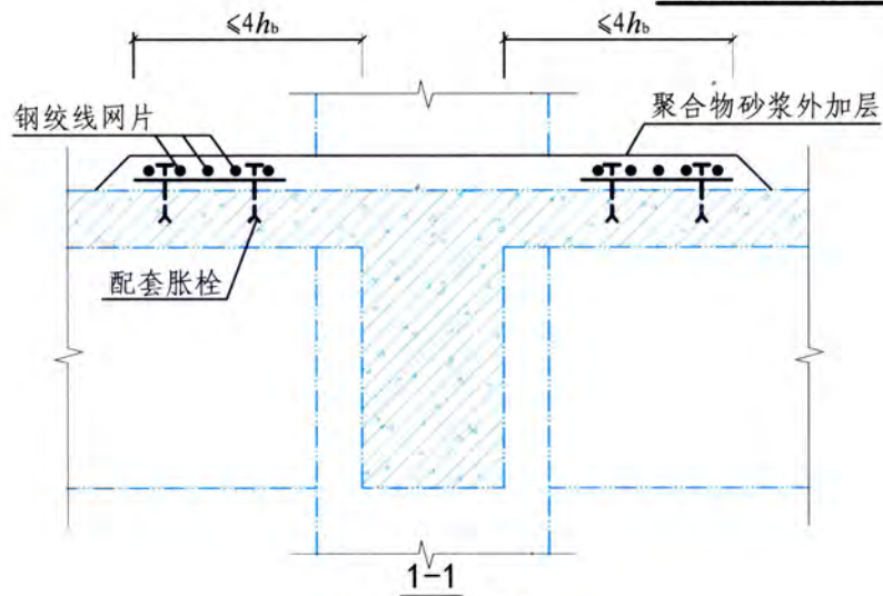
(梁顶有障碍时)
