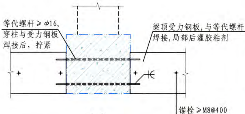
3-3
