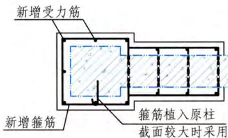
有端柱 (一)
