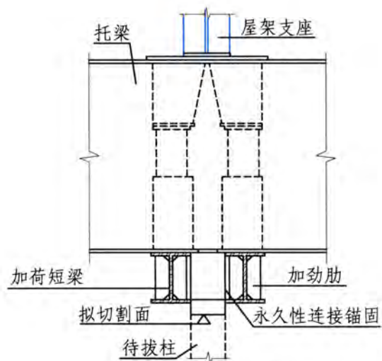
示意图(步骤3)
