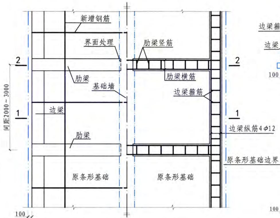
条形基础肋梁加固平面图
