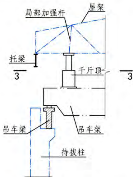
制作安装托梁(步骤3)
