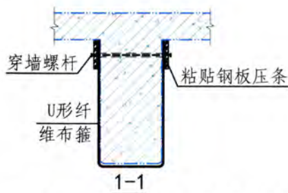
粘贴纤维布法
