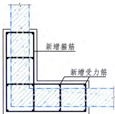
L形墙 (一)
