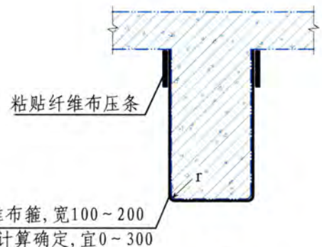
1-1 (一般U形箍)
