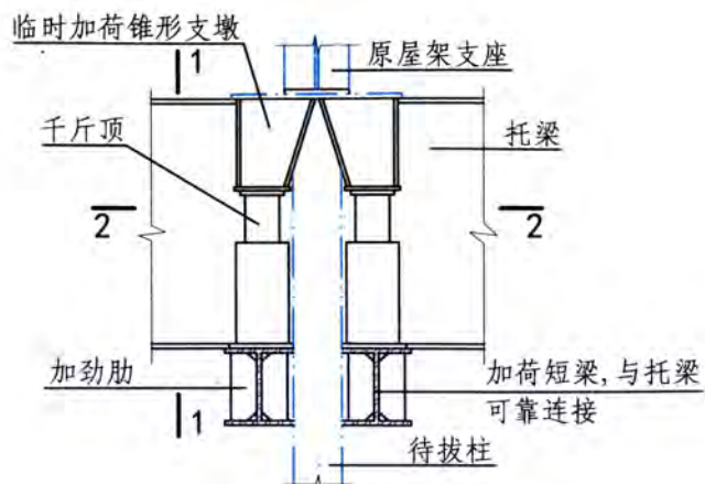
示意图(步骤2)
