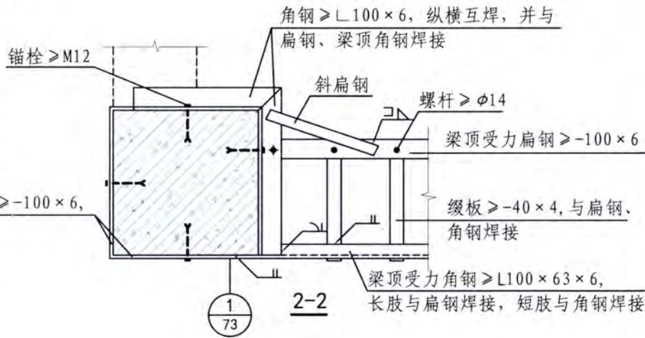
边框架梁外粘型钢加固 (型钢箍锚固)
