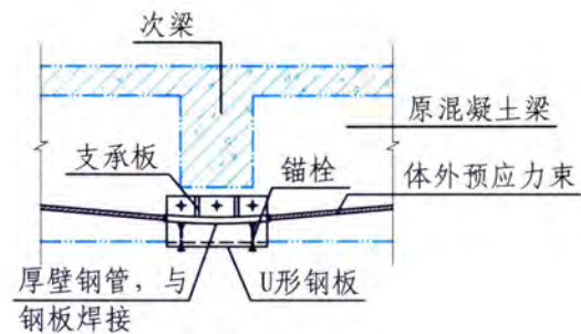
转向块4
