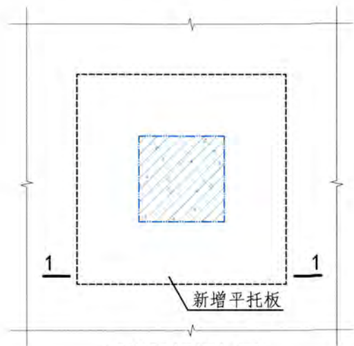
新增平托板加固
