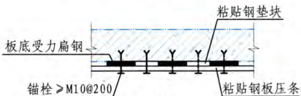
3-3
