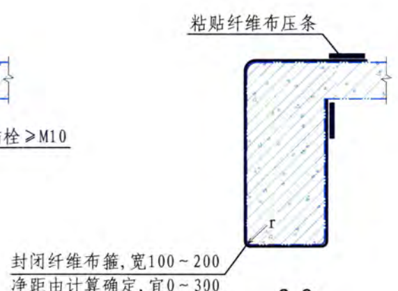
2-2 (一般U形箍)
