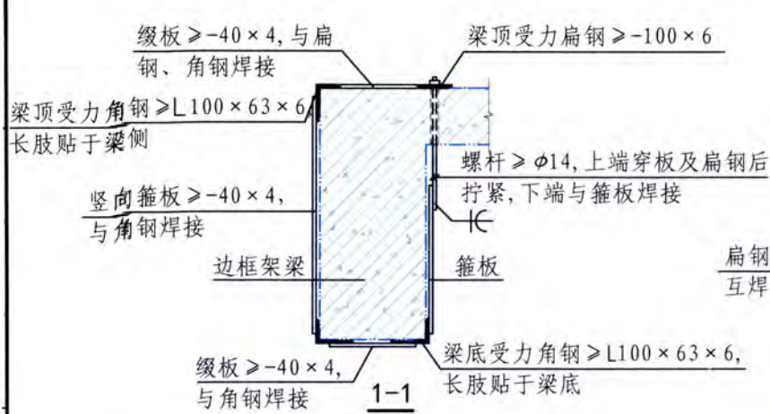
边框架梁外粘型钢加固 (型钢箍锚固)
