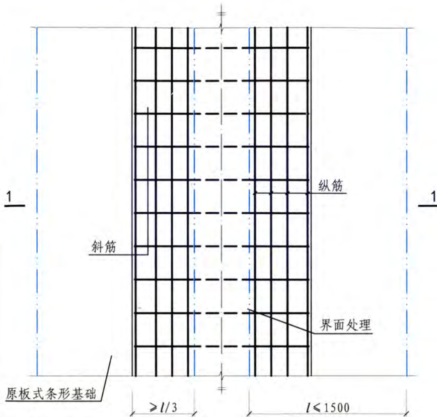
条形基础加腋加固平面图
