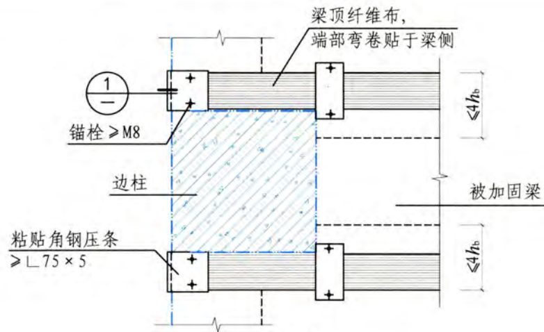
3-3 (梁顶有柱无墙时, 弯折于边梁侧锚固)
