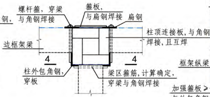
顶层边节点
