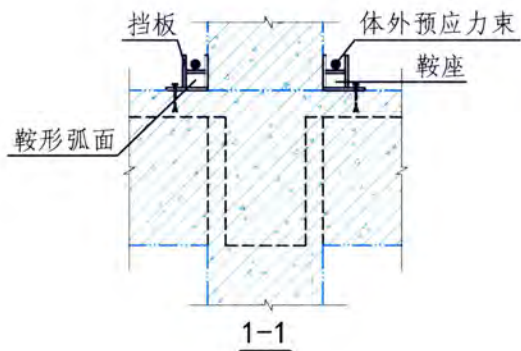
1-1 转向块1 (鞍形转向块)
