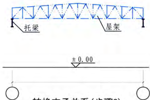
转换支承关系(步骤3)
