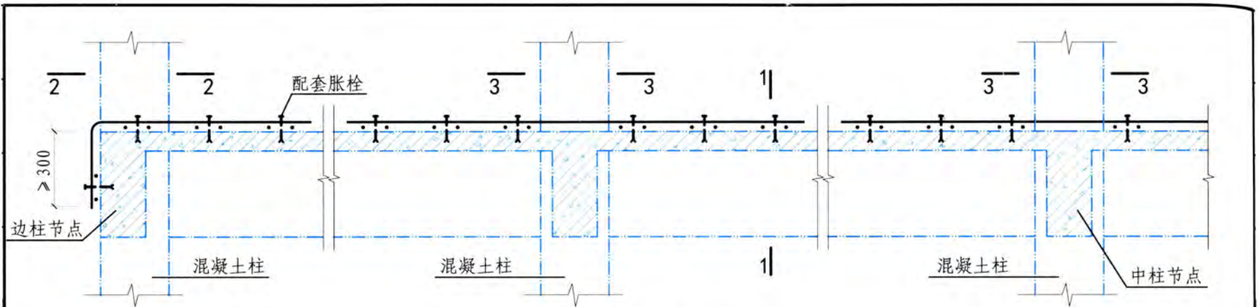
梁顶钢绞线布置示意图
