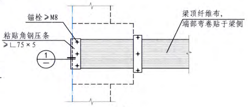
3-3 (梁顶无柱无墙时, 弯折于边梁侧锚固)
