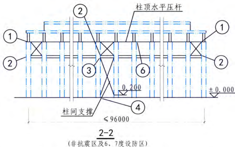
单层工业厂房有吊车情况侧向支撑布置示意图
