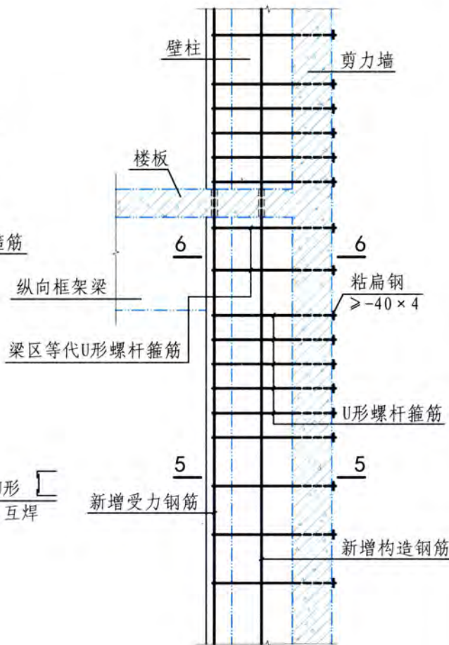
三面围套 (壁柱)
