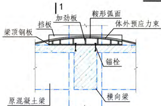
1-1 转向块1 (鞍形转向块)
