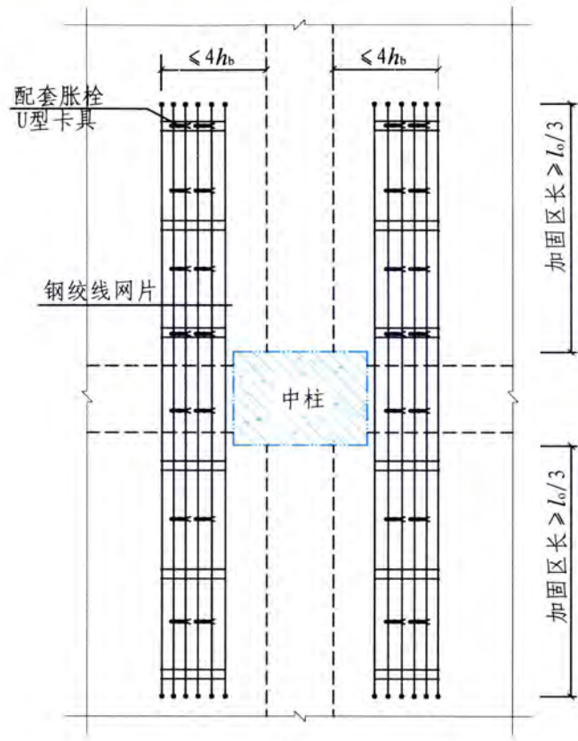
3-3 (中跨节点)
