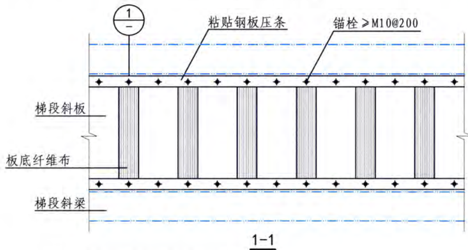
梁式楼梯梯板加固 (一)
