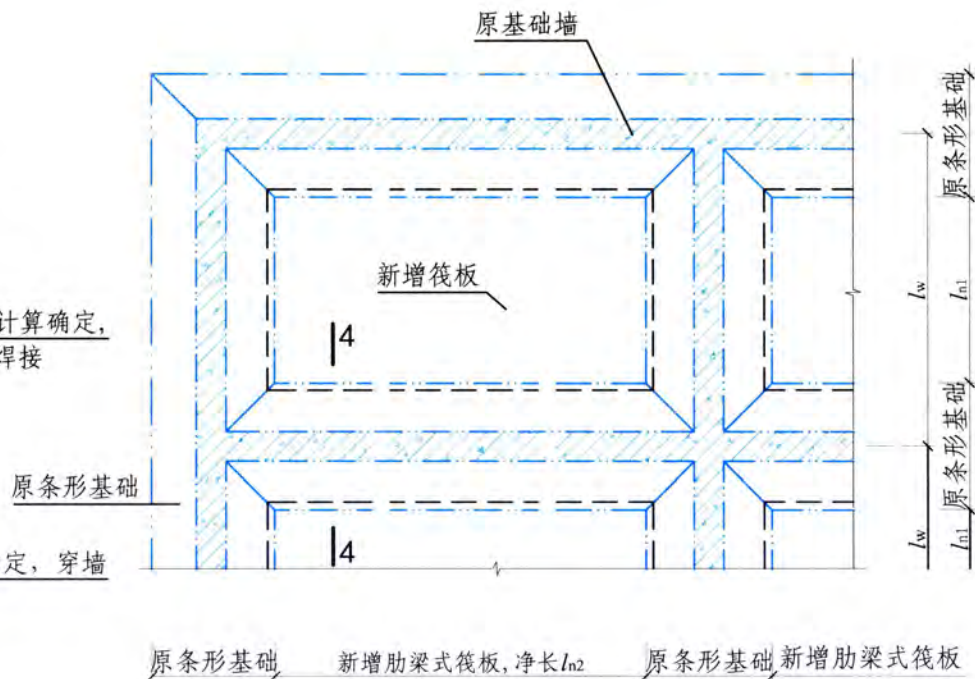
平面图
