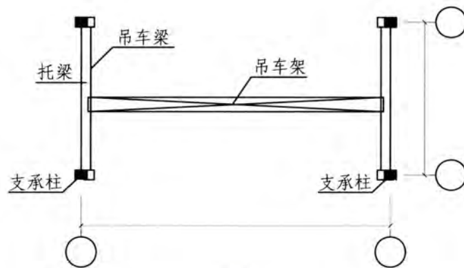
3-3
