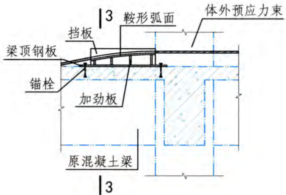
转向块3
