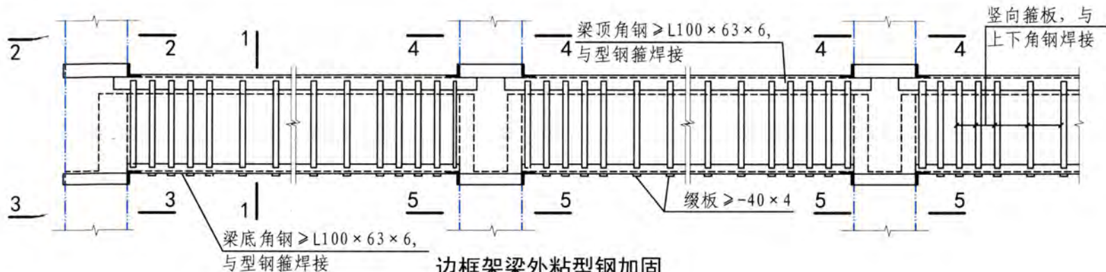
边框架梁外粘型钢加固 (型钢箍锚固)
