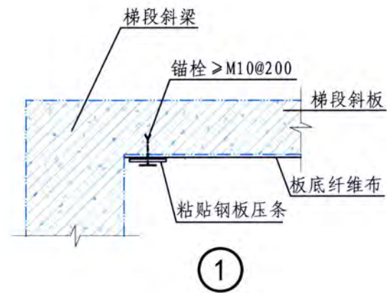
梁式楼梯梯板加固 (二)
