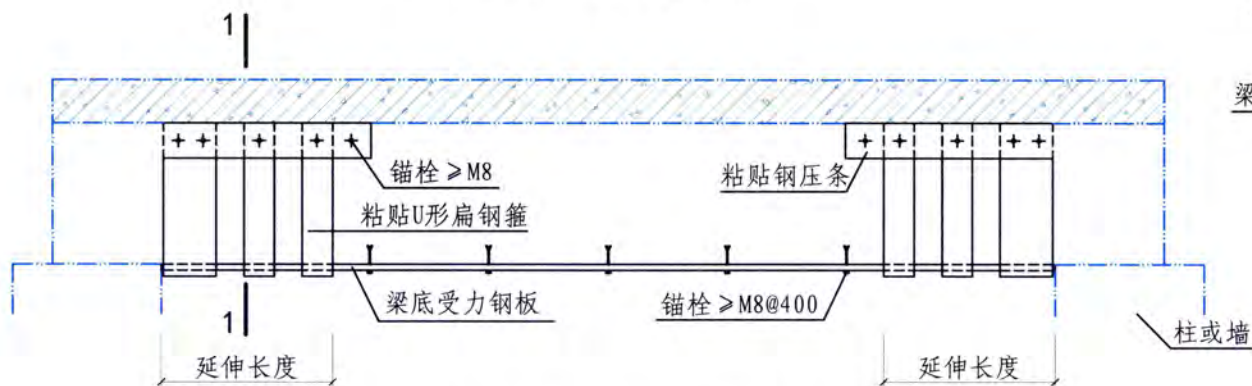
简支梁正截面粘钢加固(二)
