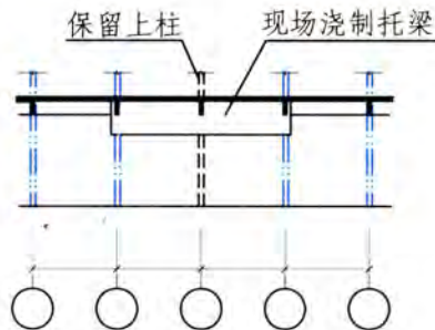
2-2 (断柱前)
