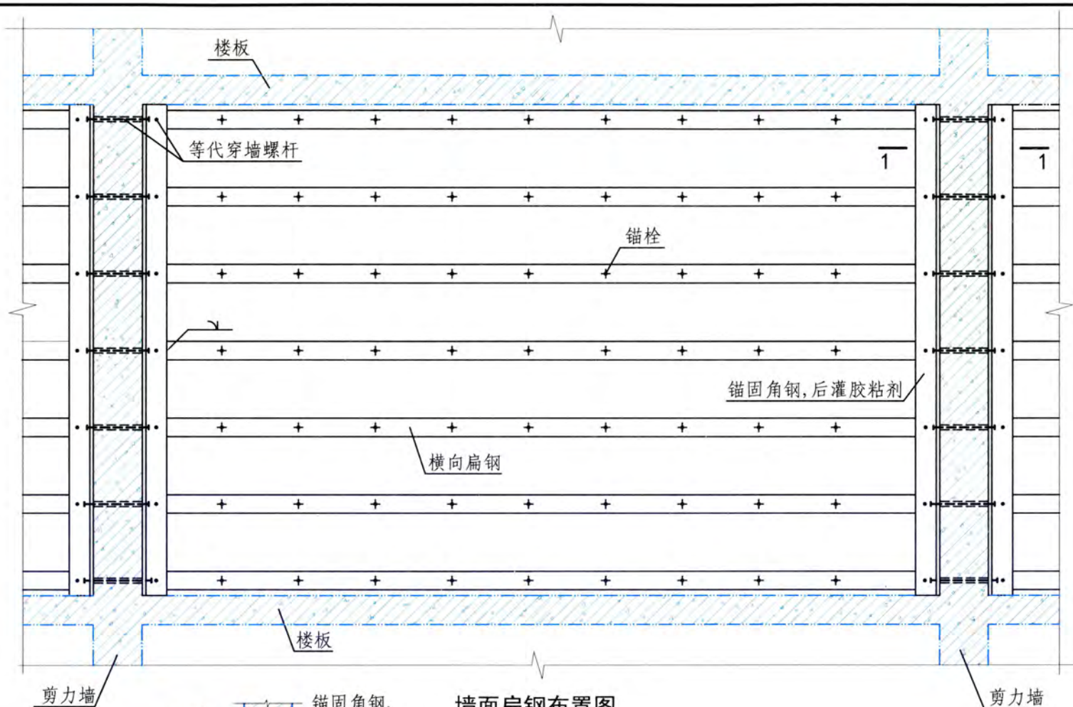
墙面扁钢布置图
