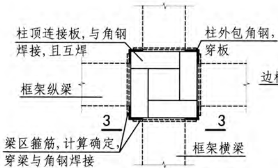
顶层中节点
