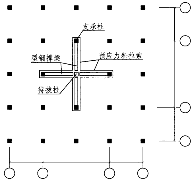
改造后结构平面图
