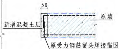
开洞部位钢筋锚固示意图
