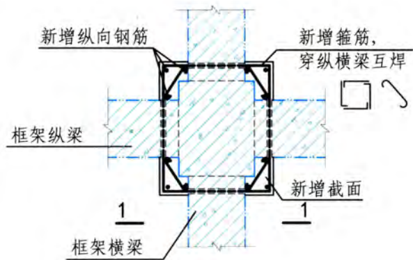
中节点
