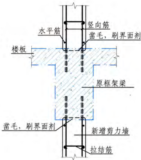
竖筋植入梁
