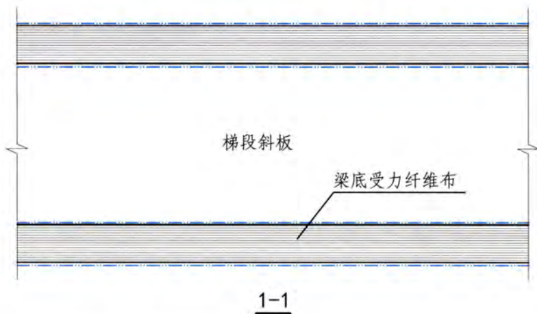
梁式楼梯梯梁加固 (一)
