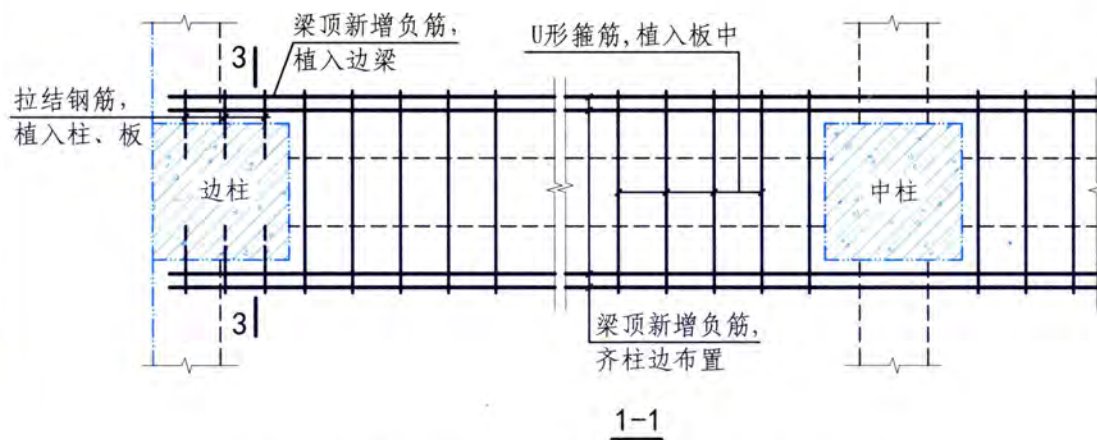
框架梁受弯承载力加固
