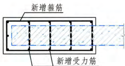
暗柱
