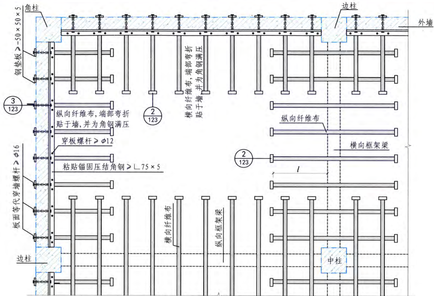
有外墙时板面纤维布置
